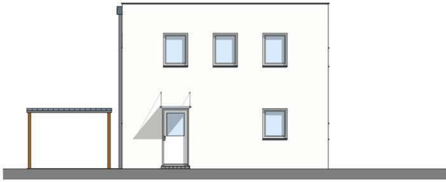
Nordansicht
