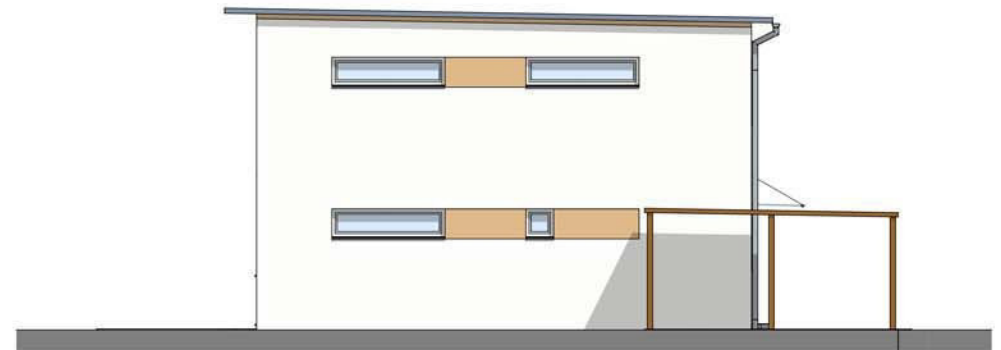
Ostansicht
