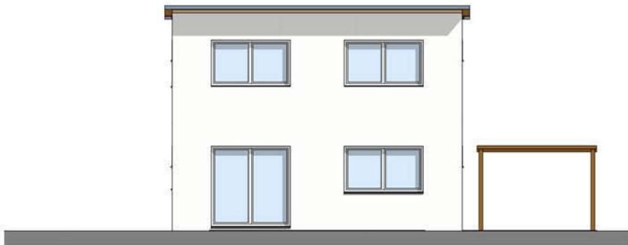
Südansicht
