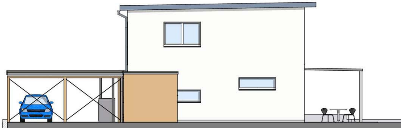
Westansicht
