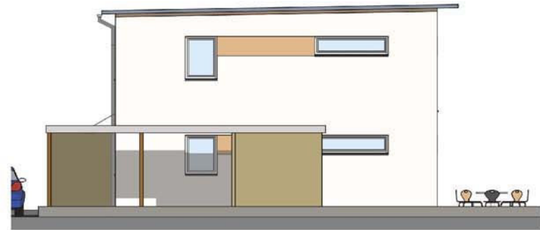
Westansicht
